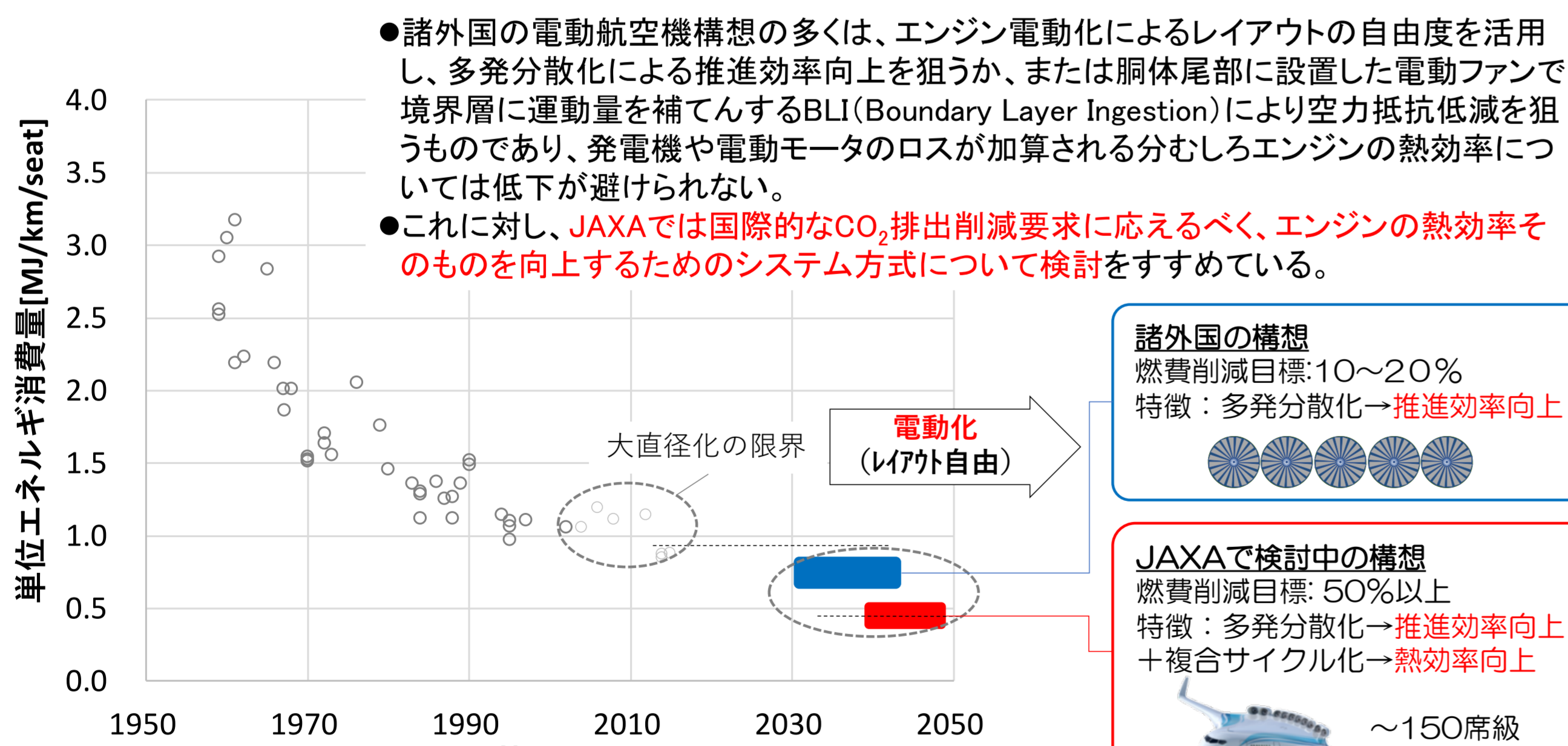
航空機の単位エネルギー消費量の推移と将来目標
