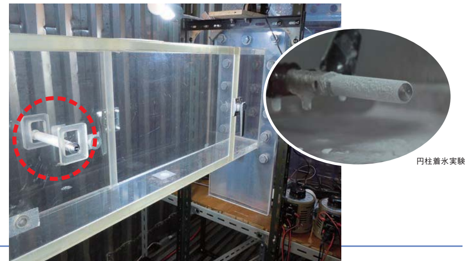
神奈川工科大学の着氷風洞
