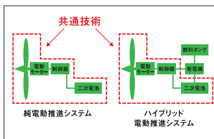
電動航空機のシステム構成
