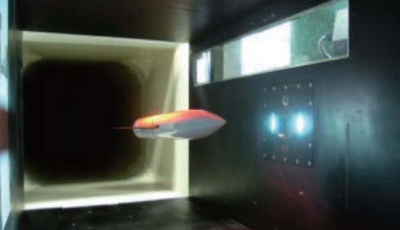
航空機の標準模型 (AGARD-B模型)の実験写真
