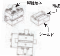
極低温ロケット燃料配管、ボイドメーター(2個)、極低温ボイドメーターの概要
