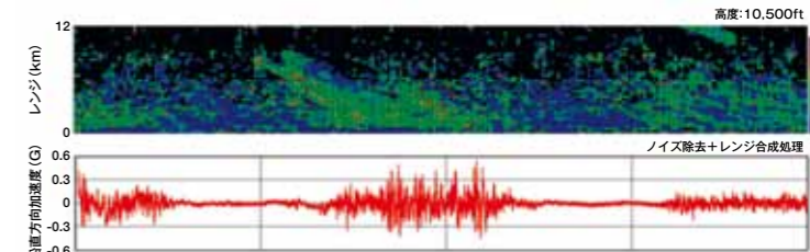
図2 計測された晴天乱気流のデータ
