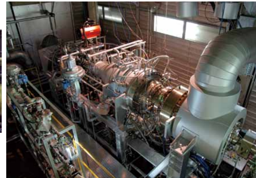
環状燃焼器試験設備 ジェットエンジン燃焼器全体の試験を行う。
