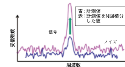
図1 N回積分によるS/N比の改善
