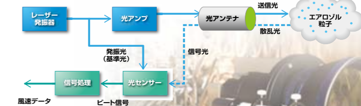
図3 ヘテロダイン方式
