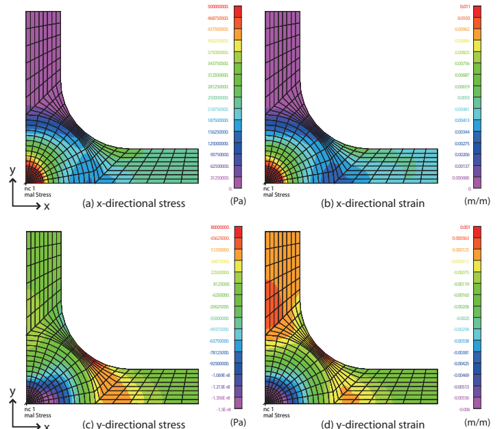
図3 単軸負荷での十字型試験片の応力(左)とひずみの分布(右)。一方方向からの荷重によって、その方向以外にも応力やひずみが生じていることが分かる。
