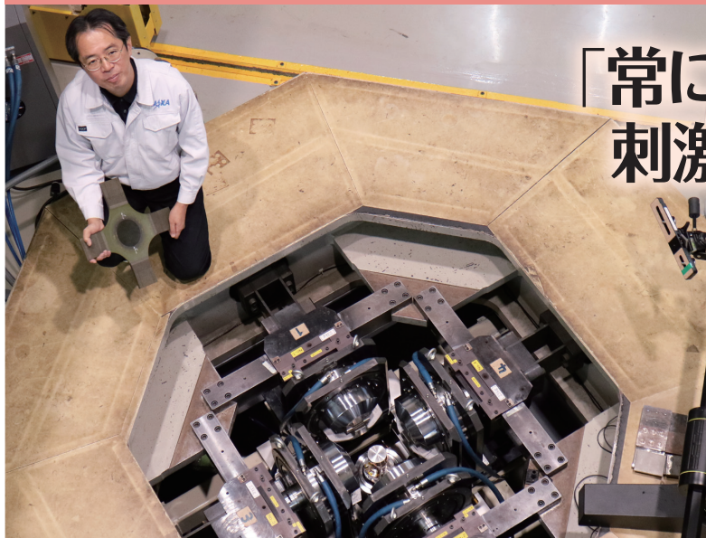
二軸疲労試験機の上で、十字型の構造試験用試験片を手に。
