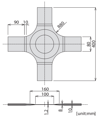
図2 試験片形状の例。400mm角の試験片が標準的な試験片の大きさ。標準的な試験片の測定エリアの厚みは、1mmから2mm程度。
