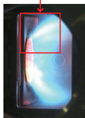
「高温高圧燃焼試験設備での燃焼振動実験データ(燃焼器入口圧力:7気圧、入口温度:760K)」 高速OH-PLIFによって、1万分の1秒間隔で撮影した燃焼振動発生時の火炎断層写真。 F-Gに見られる火炎の逆流が周期的に発生している。
