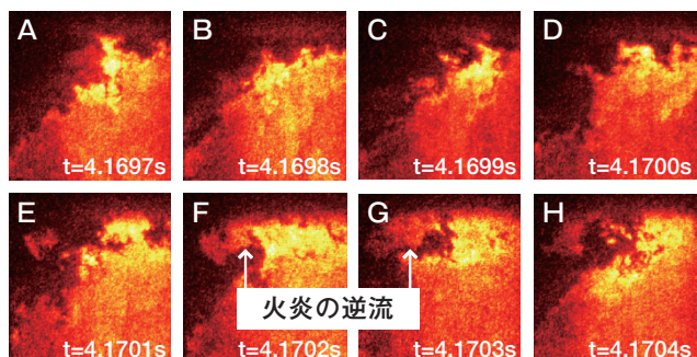
「高温高圧燃焼試験設備での燃焼振動実験データ(燃焼器入口圧力:7気圧、入口温度:760K)」 高速OH-PLIFによって、1万分の1秒間隔で撮影した燃焼振動発生時の火炎断層写真。 F-Gに見られる火炎の逆流が周期的に発生している。
