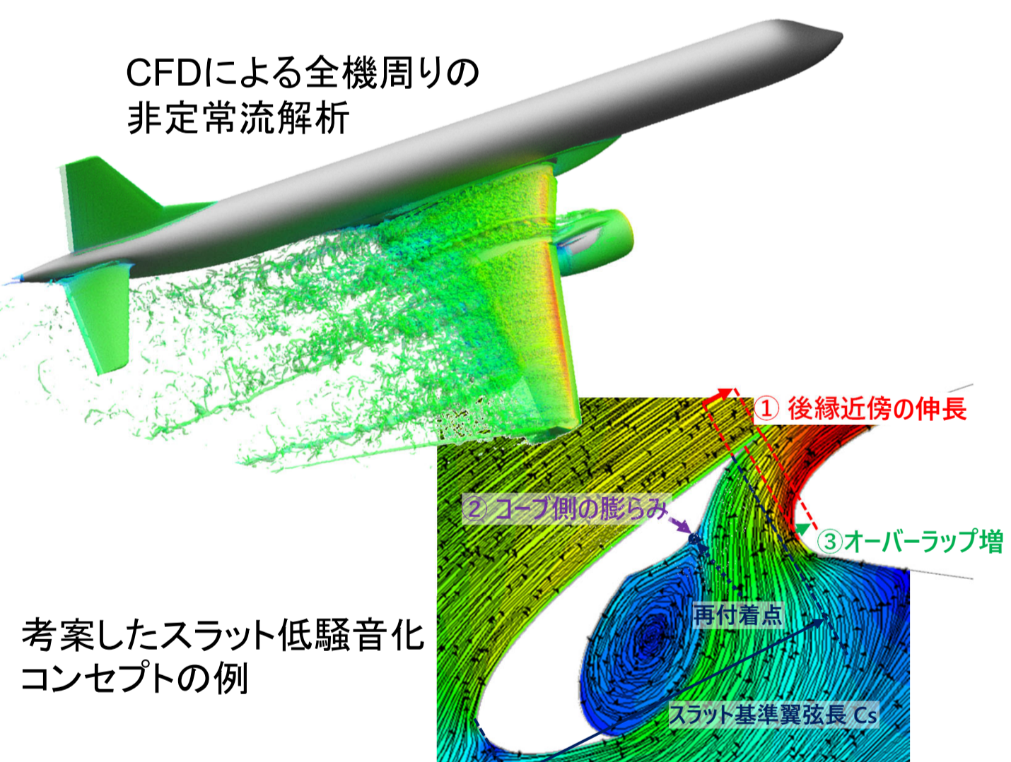
CFDを活用した低騒音化設計
