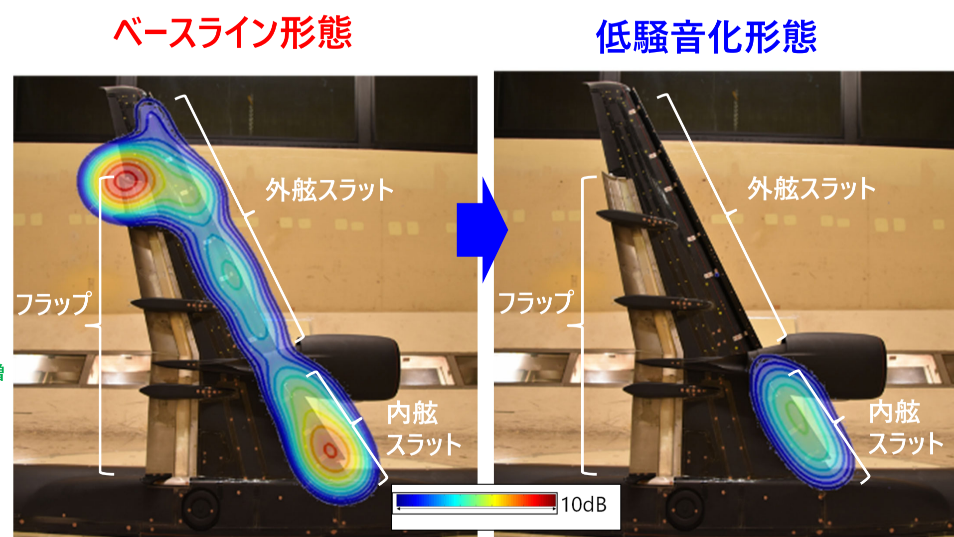
風洞試験による低騒音化前後の音源分布比較
