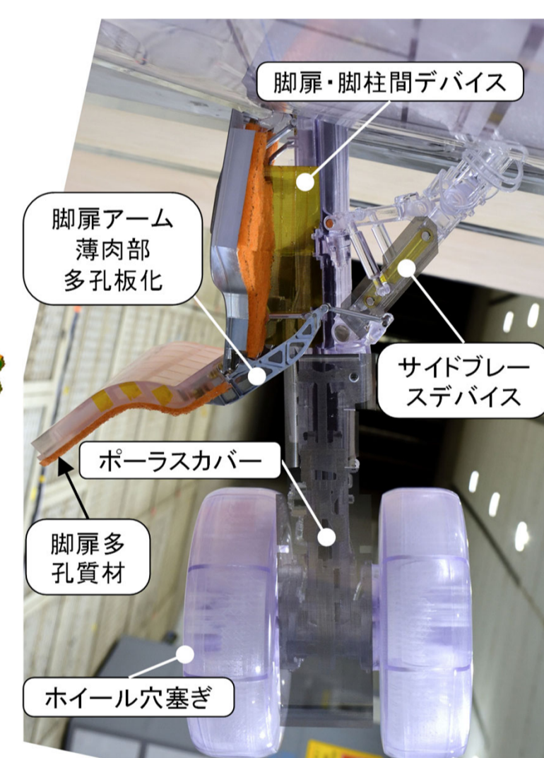
低騒音化形態 (上流側から)
