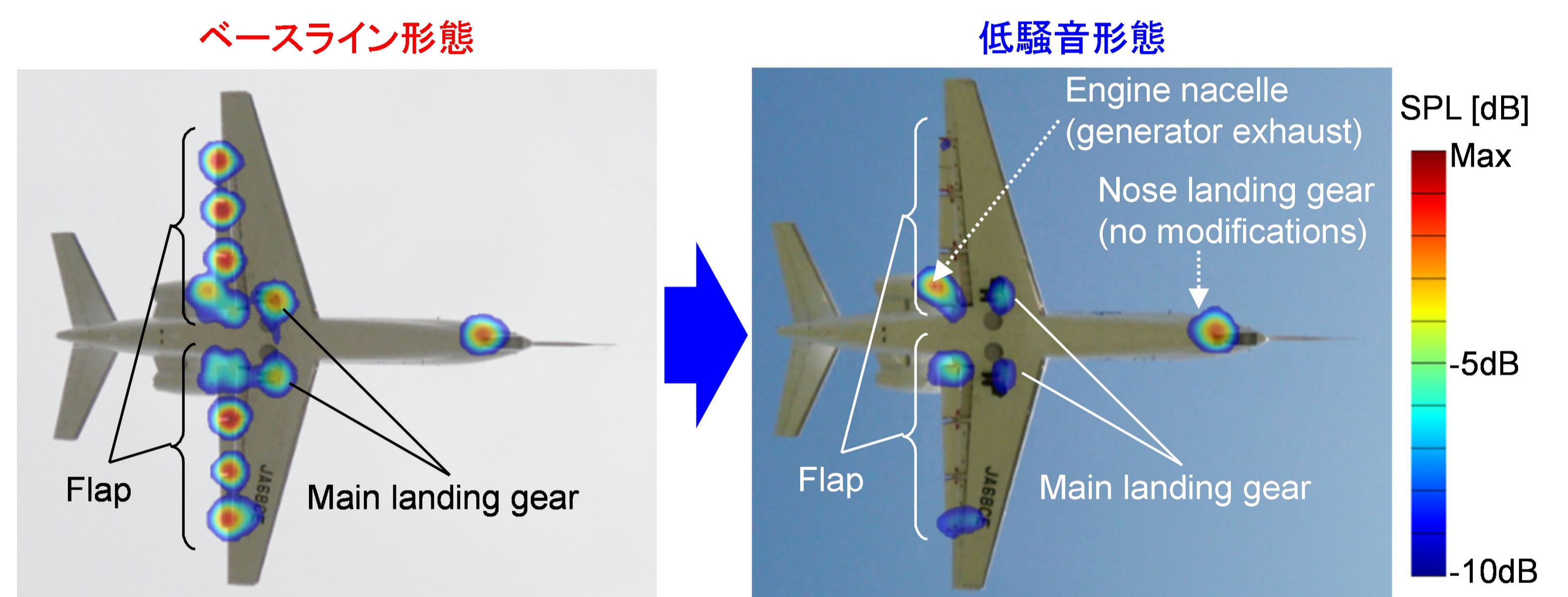
低騒音化前後のJAXA実験機「飛翔」の1 kHzでの音源分布
