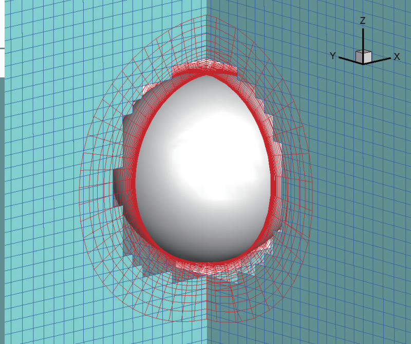
FaSTAR-Moveで解析に用いる重合格子の例。
