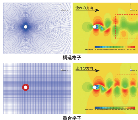
図 流れの中にある円柱を構造格子(上)と重合格子(下)で解析した場合の比較。構造格子では物体から離れた場所(点線で囲った部分)の解像度が粗くなってしまいが、重合格子であれば高い解像度で解析でき、流れの様子が明確に分かる(左図:計算格子 右図:マッシュ数分布)。
