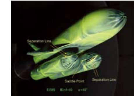
最使用宇宙往還機オイルフロー試験 Oil Flow Test of Future Re-usable Space Transport
