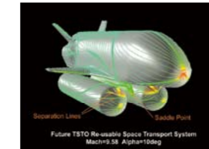
再使用宇宙往還機オイルフロー数値シミュレーション CFD of Future Re-usable Space Transport
