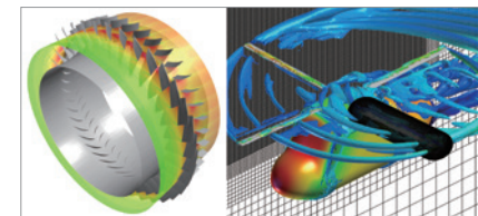
エンジン圧縮機 翼列解析および ヘリコプタ胴体／ ロータ干渉解析
