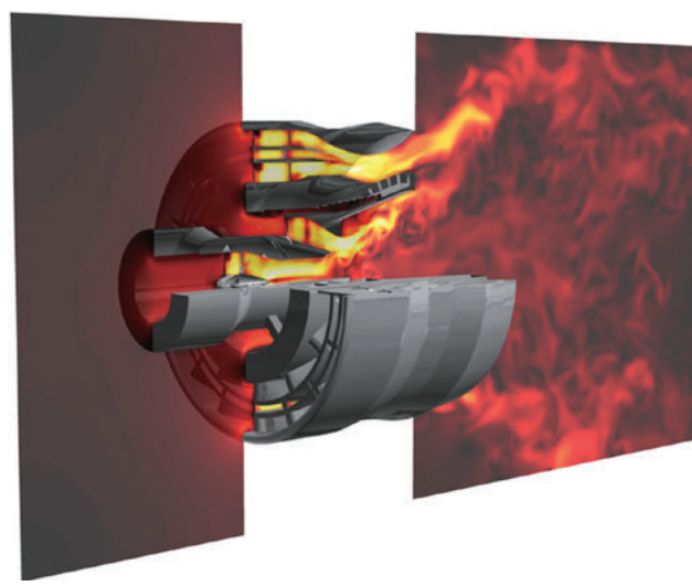
エンジン燃焼解析ソフトウェア「HINOCA」による 航空エンジン燃料ノズルの解析結果のマッハ数分布
