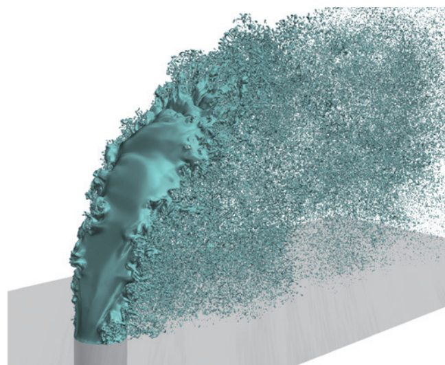
燃料ジェット微粒化過程の現象解明
